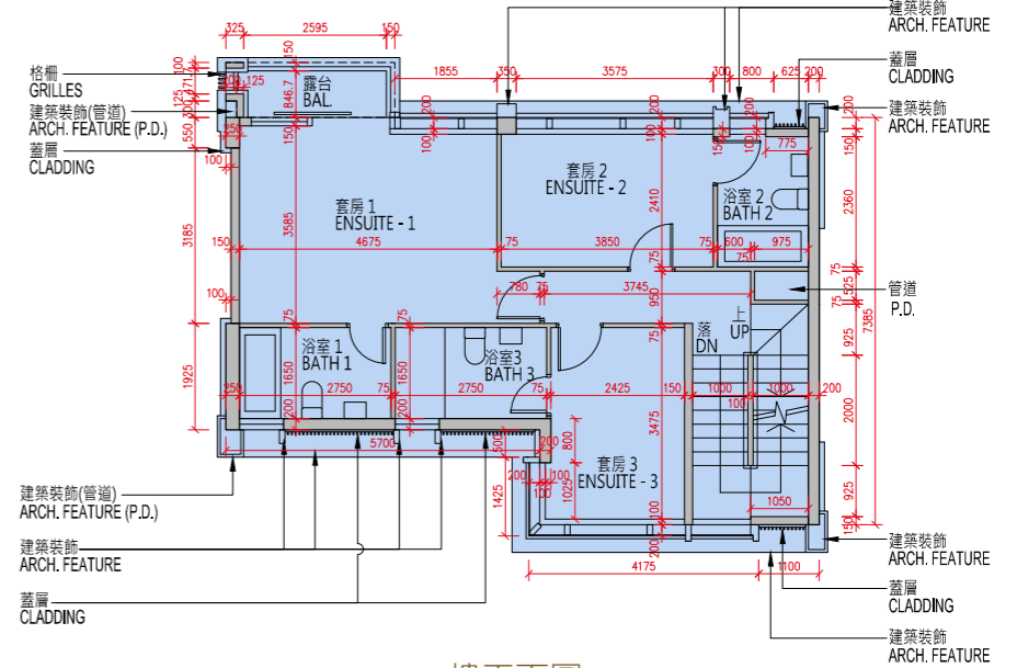
一樓平面圖 1/F PLAN
