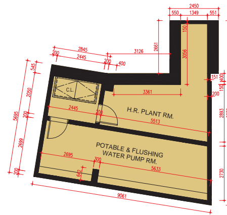
M/E ROOM FLOOR PLAN 機房平面圖
