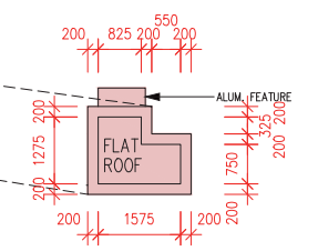
TOP ROOF PART PLAN 天台頂層局部平面圖
