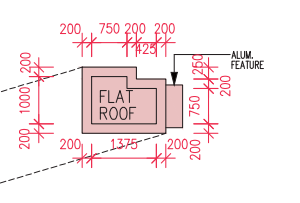
TOP ROOF PART PLAN 天台頂層局部平面圖
