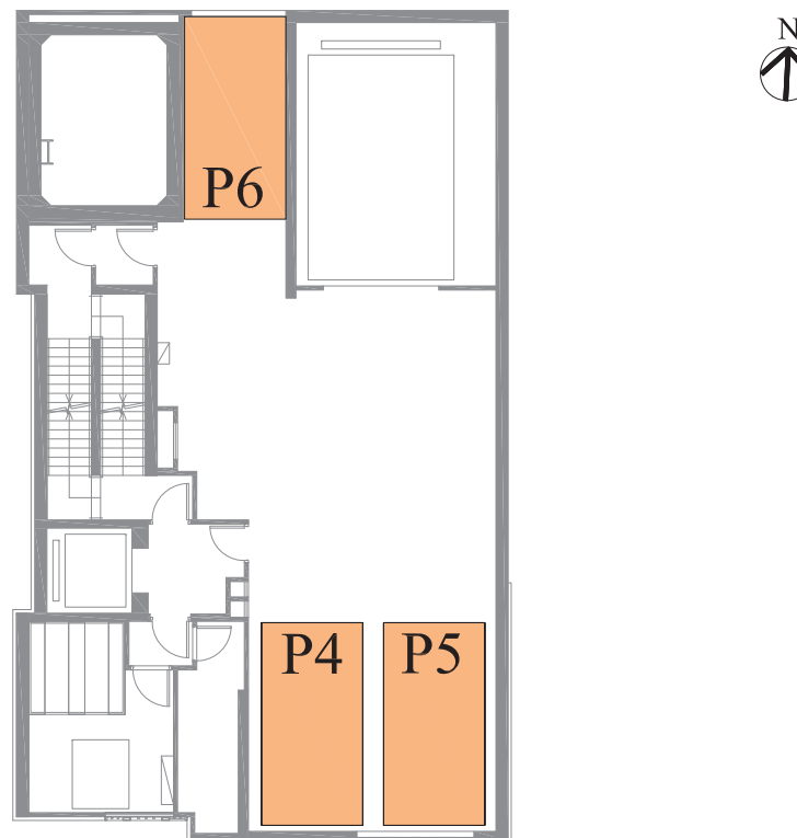
2/F CAR PARK PLAN 2樓停車場平面圖
