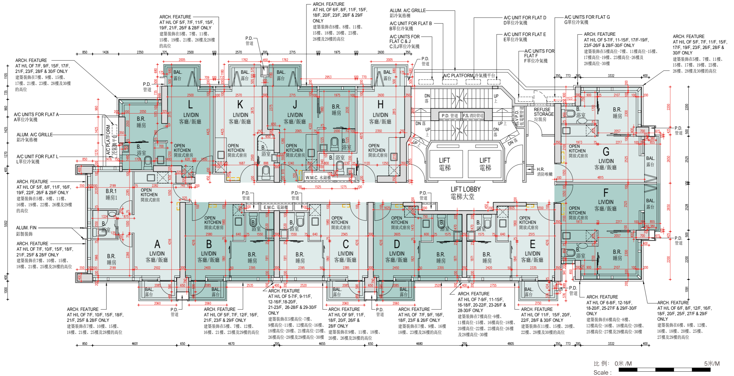
6樓-12樓、15樓-23樓及25樓-30樓平面圖 6/F-12/F, 15/F-23/F & 25/F-30/F Floor Plan
