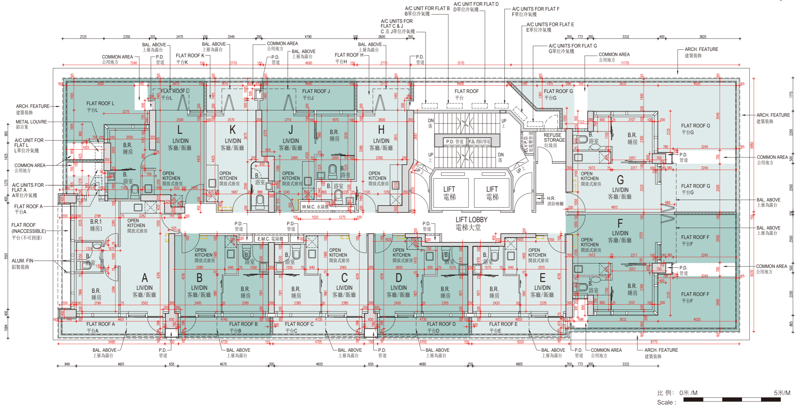
5樓平面圖 5/F Floor Plan
