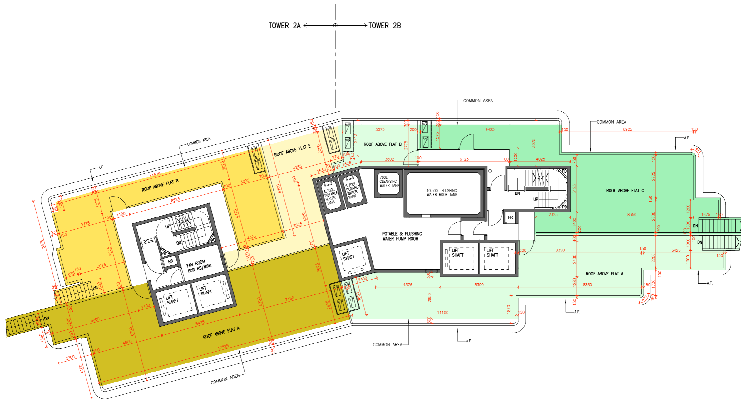
第2座天台平面圖 Tower 2, Roof Floor Plan
