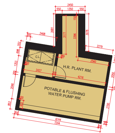
M/E ROOM FLOOR PLAN 機房平面圖
