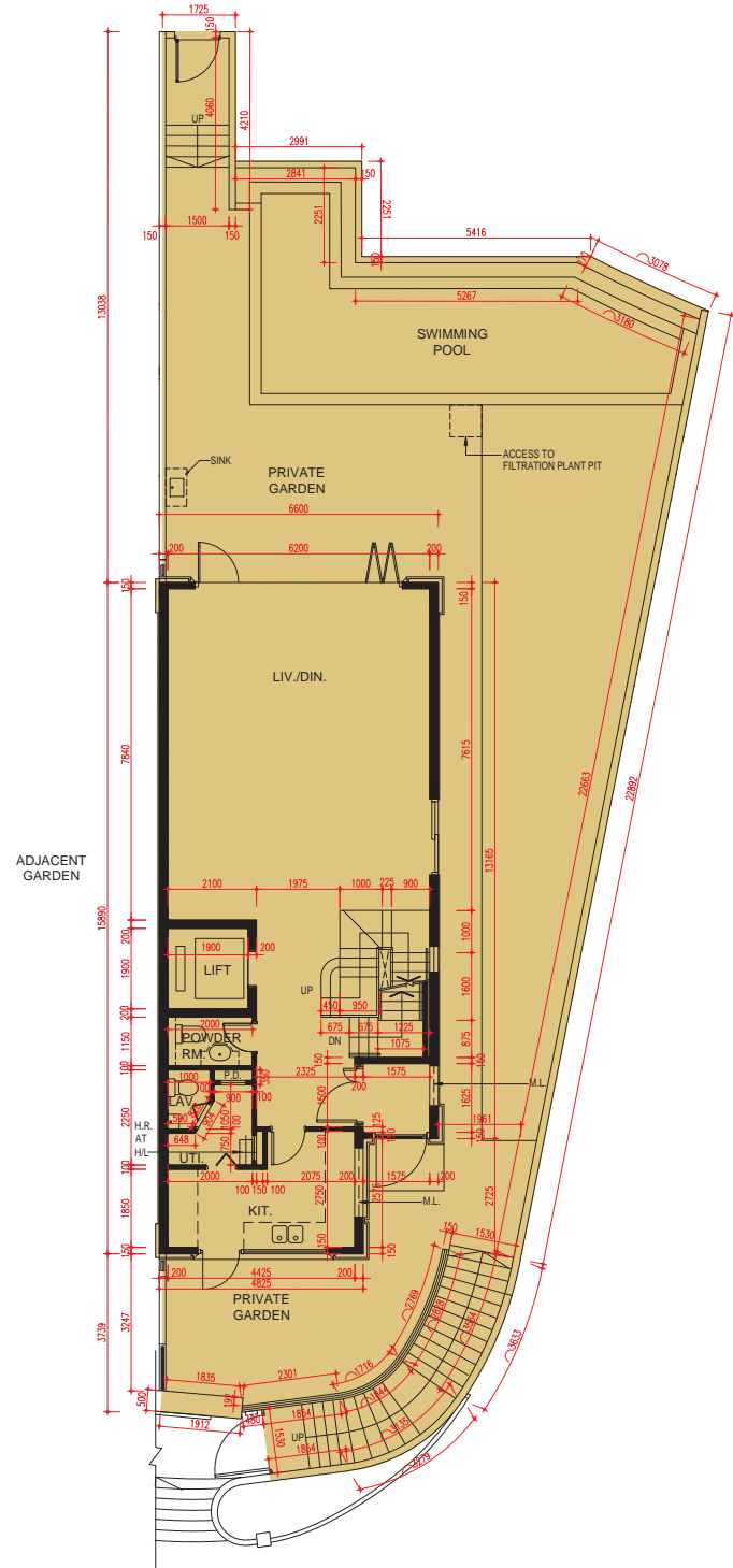
G/F FLOOR PLAN 地下平面圖
