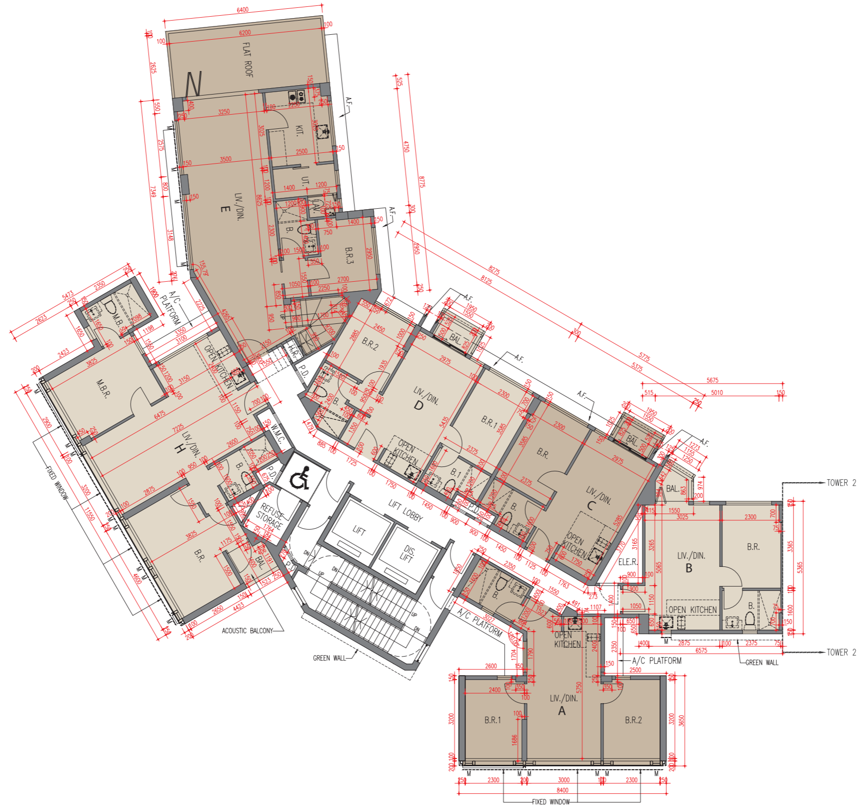
9樓平面圖 9/F Plan
