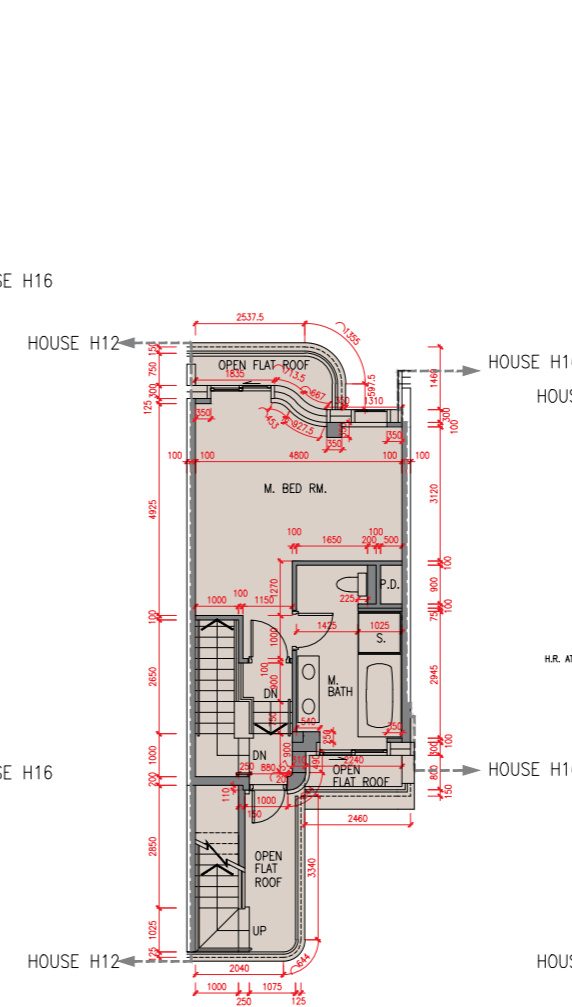
2樓平面圖 2/F Plan
