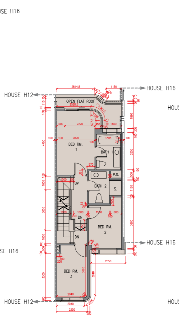
1樓平面圖 1/F Plan
