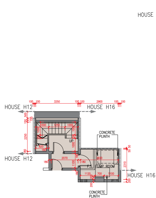
地庫平面圖 B/F Plan
