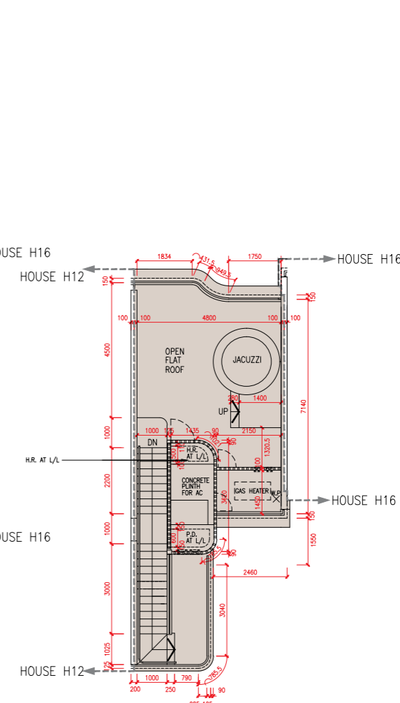
天台平面圖 Roof Plan
