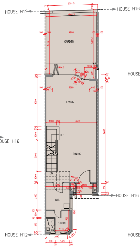
地下平面圖 G/F Plan
