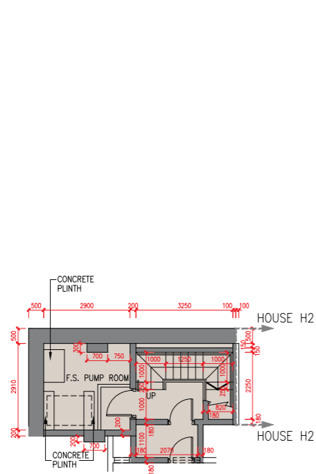
地庫平面圖 B/F Plan
