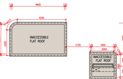
頂層天台平面圖 Top Roof Plan
